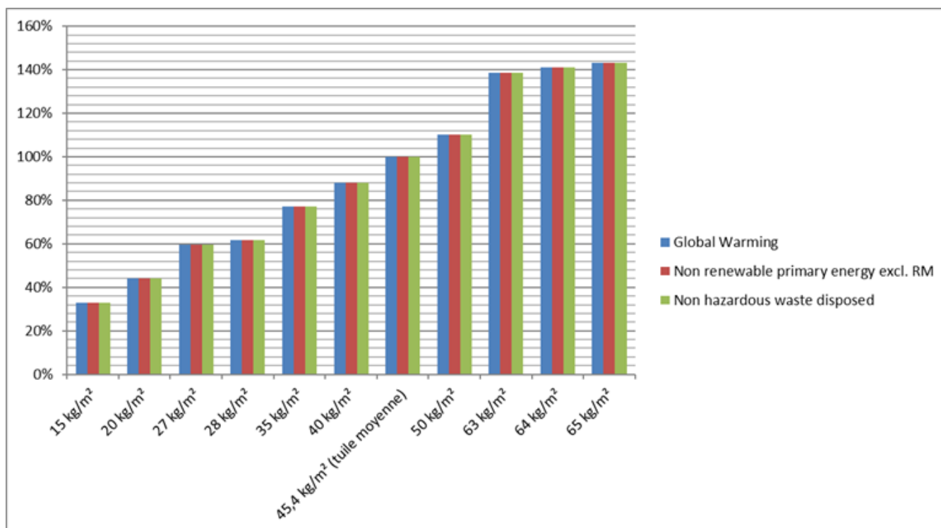
Graphique illustrant la variabilité des résultats d'impacts environnementaux sur 3 indicateurs en fonction de la variation de la masse de tuiles à emboîtement au mètre carré
