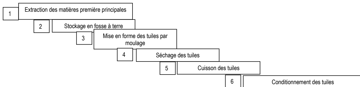
Schéma décrivant le procédé classique de fabrication des tuiles à emboîtement
